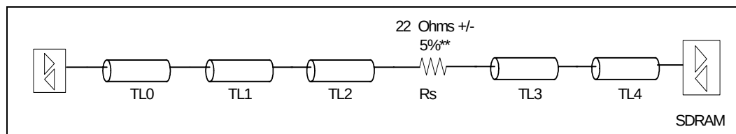
Figure 55. DDR II 400 Embedded DQ Topology
