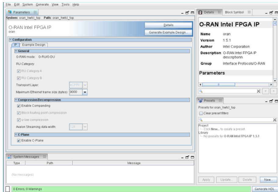
Figure 4. O-RAN IP Parameter Editor
