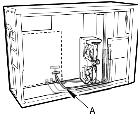
Figure 13. Passage du câble du lecteur de disquettes
