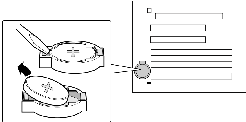
Figure 23. Remplacement de la pile de secours
