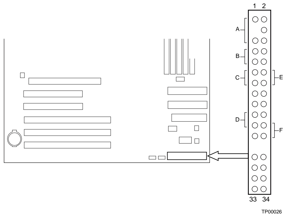
Figure 29. Emplacement de la connexion du support de panneau avant
