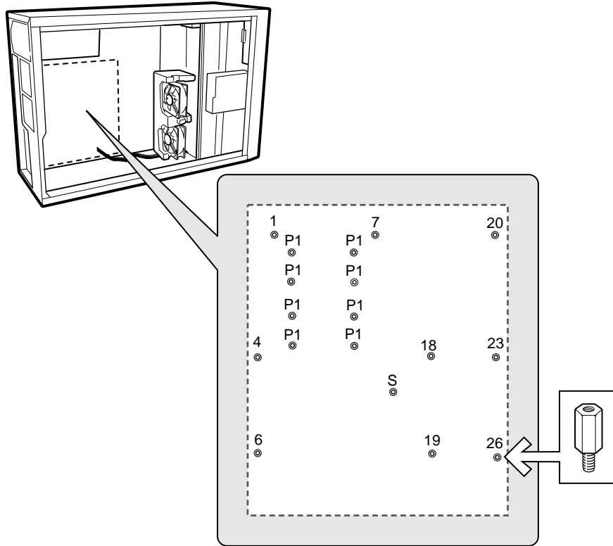
Figure 6. Configuration des isolateurs du châssis
