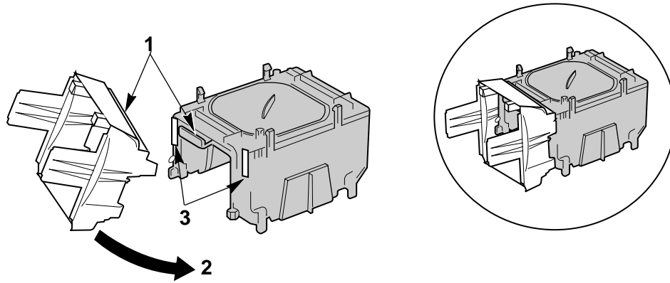
Figure 19. Fixation du boîtier du ventilateur sur le tunnel
