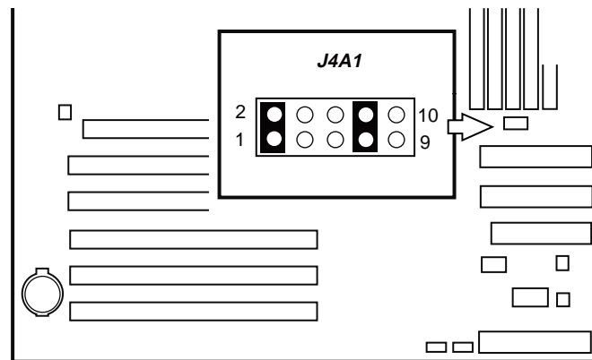
Figure 26. Cavalier de récupération du mot de passe
