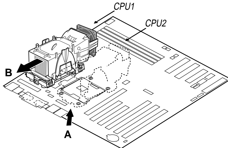
Figure 22. Processeur et tunnel processeur installés
