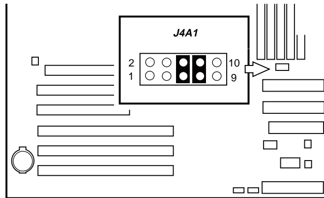
Figure 27. Cavalier de récupération du CMOS
