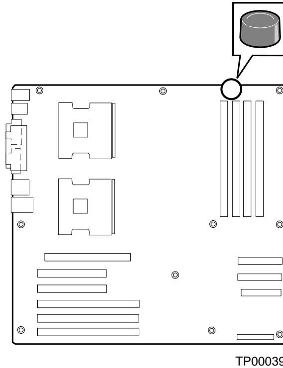
Figure 7. Installation du Tampon caoutchouc
