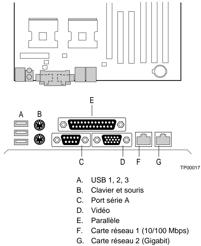
Figure 2. Connecteurs du panneau arrière
