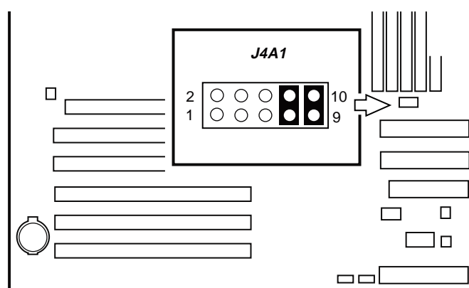
Figure 28. Emplacement des cavaliers de configuration
