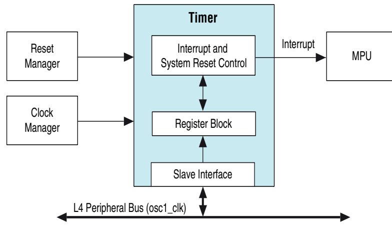
图 23 - 1. 计时器结构图
