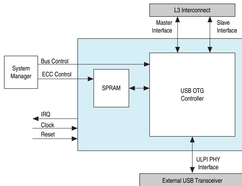
图 18-1. USB OTG 控制器系统集成
