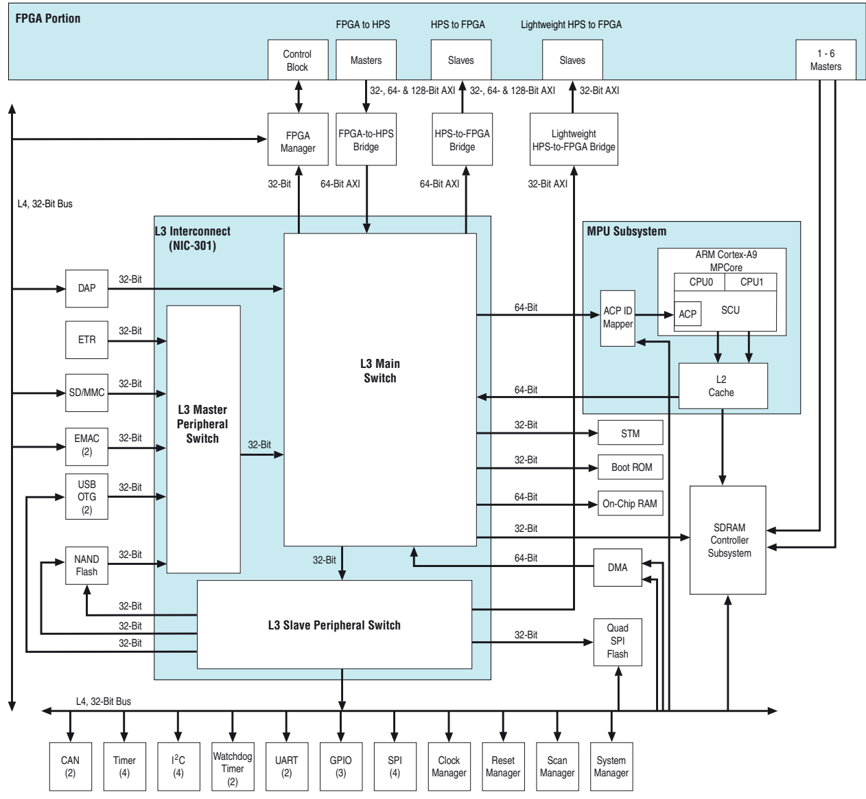
图 1-2. HPS 结构图
