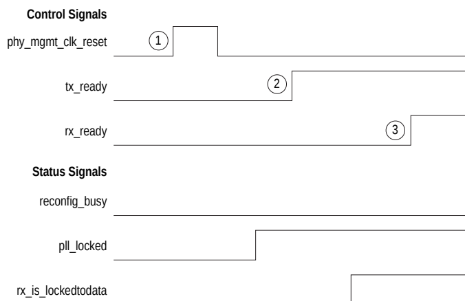
图3-3: 器件操作期间使用嵌入式复位控制器的复位流程时序图
