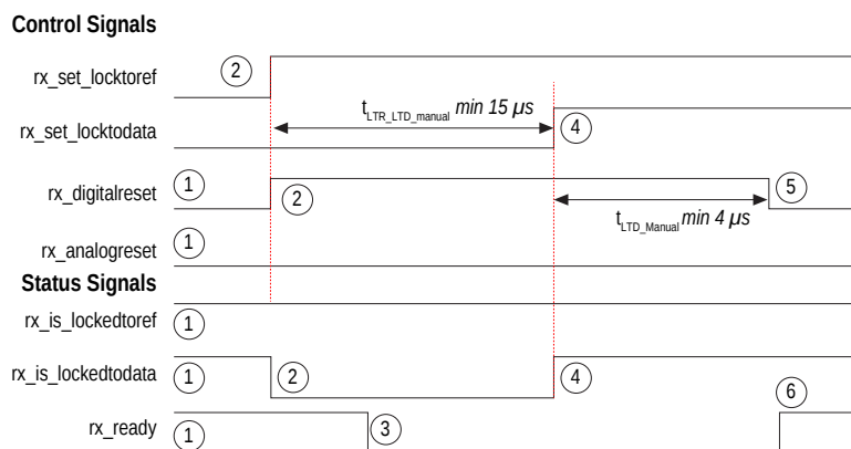
图3-9: CDR处在手动锁定模式时，收发器的复位流程时序图
