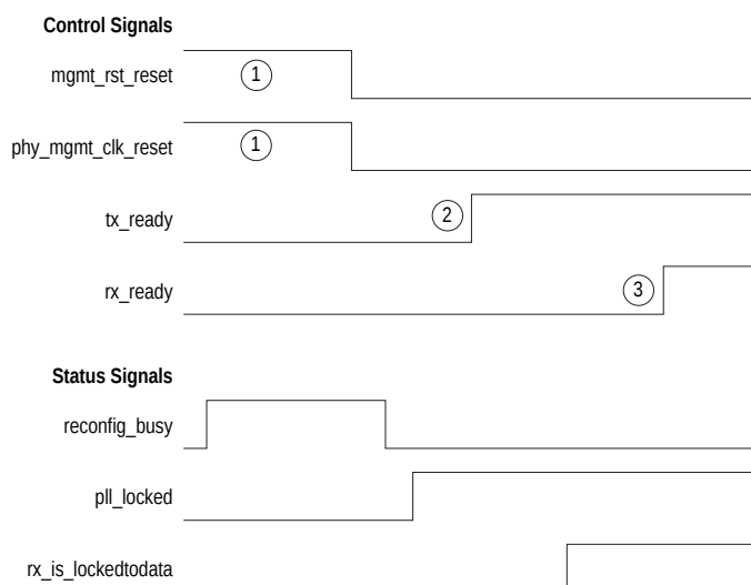
图3-2: 在器件上电期间，使用嵌入式复位控制器的复位流程时序图
