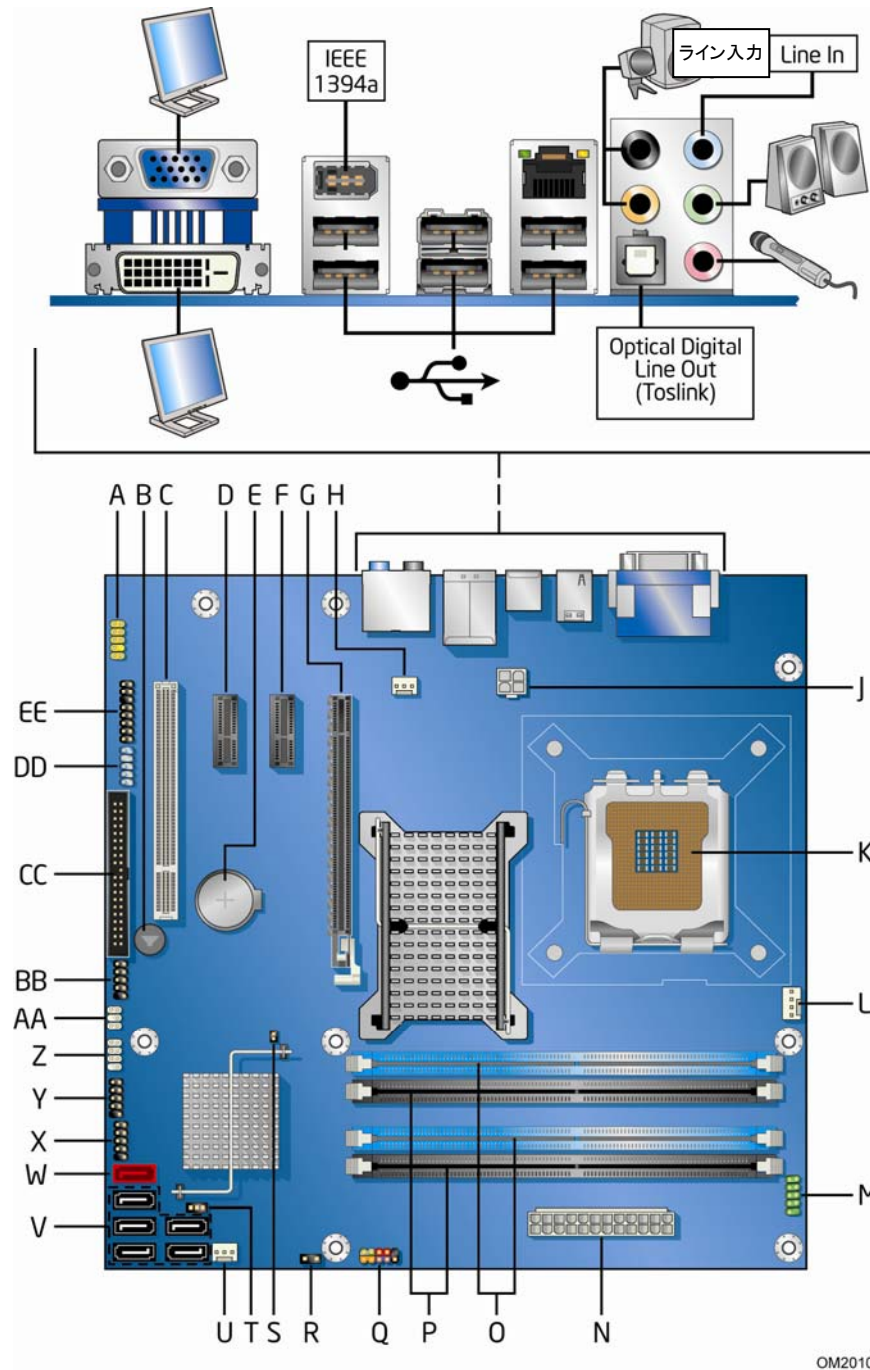
図 1. デスクトップ・ボード DG33TL のコンポーネント
